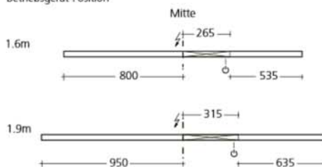
Pendel-Position Betriebsgerät-Position
